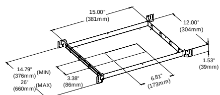
TRIM & TRIMLESS AT/IC Box: 41951-019 IC Box: 41950-012
